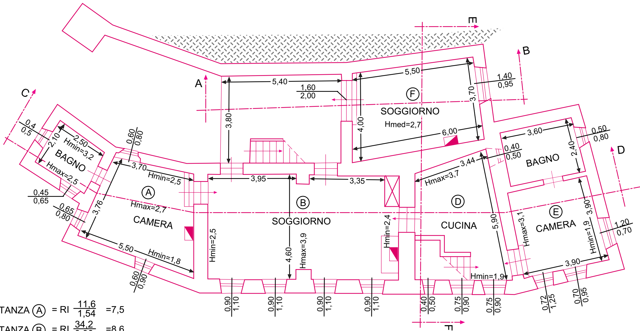
PIANTA PIANO TERRA FUTURO
