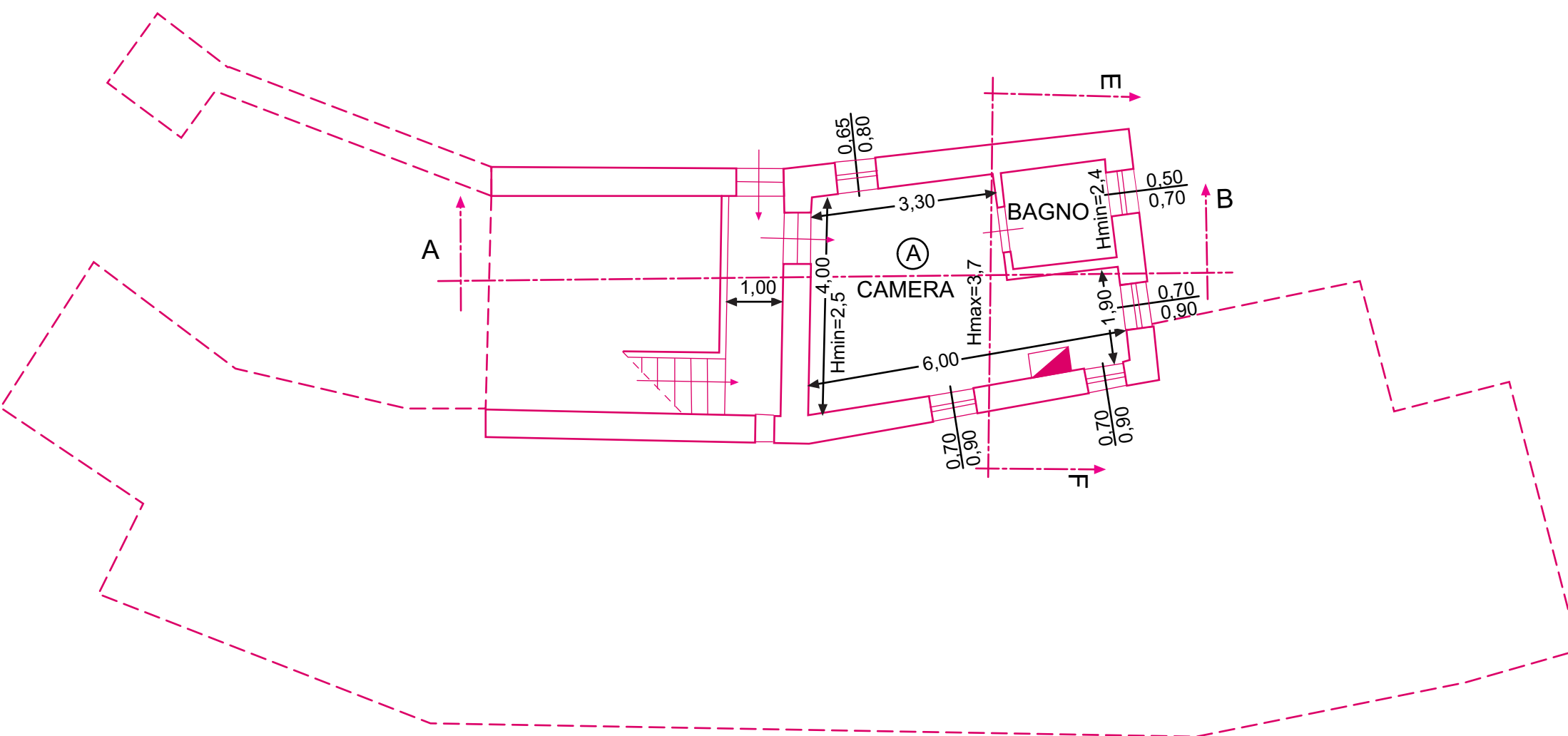
PIANTA PIANO PRIMO FUTURO
